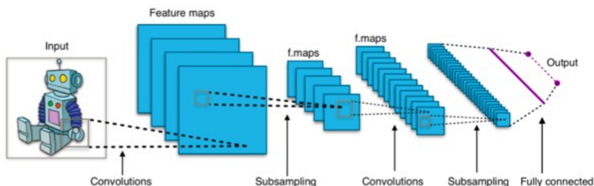
Figure 3 : Architecture standard d'un réseau convolutif 16
