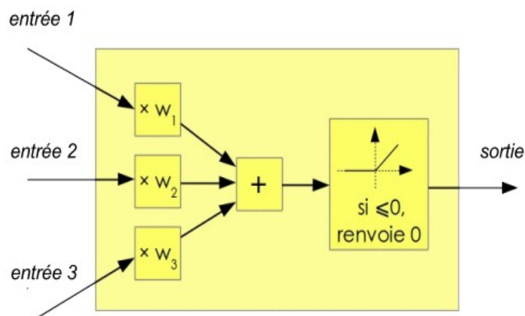
Figure 1 : Le neurone formel de McCulloch et Pitts est un modèle mathématique très simple dérivé d'une analyse de la réalité biologique (Michel Blancard 11 )
